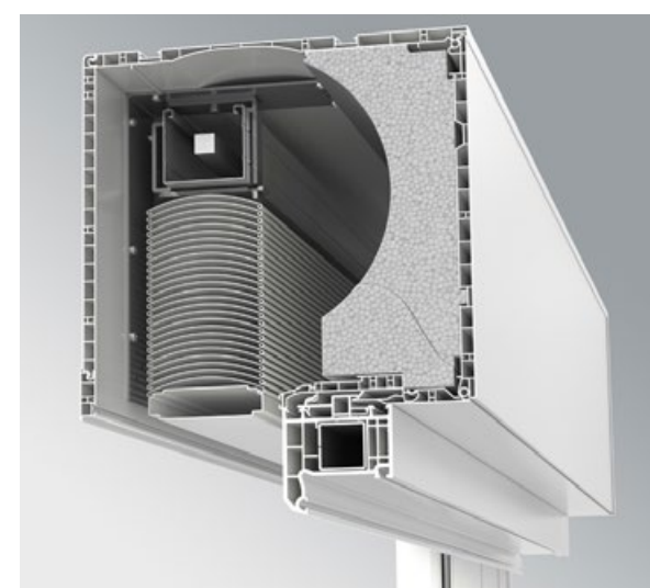
Zsaluzia tokrendszer
